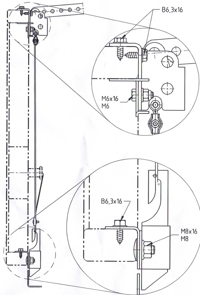
Montagezeichnung für Verriegelungsset mittig plan de montage pour unité de verrouillage centrée 150451-01-6-50
